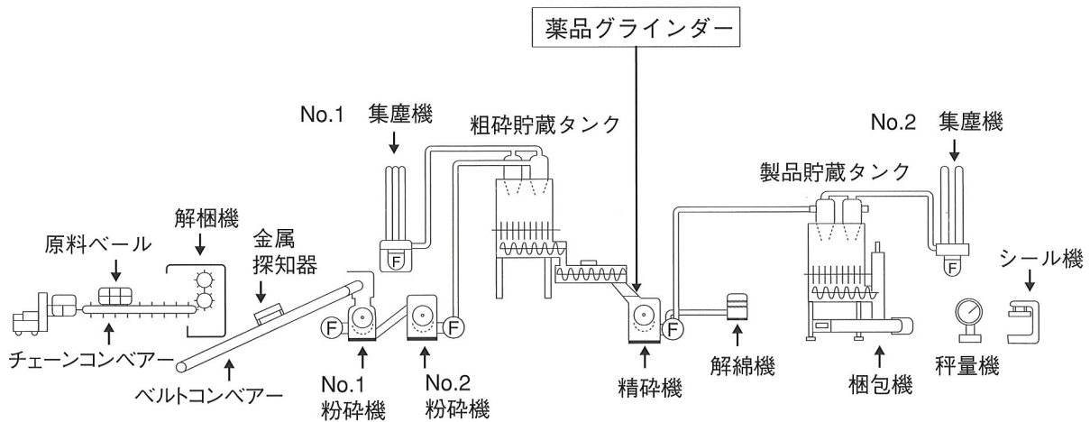
セルローズファイバーの製造工程の例
